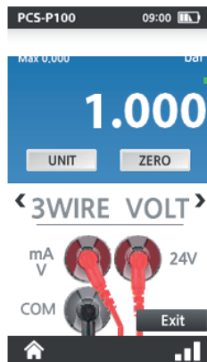
ヘルプ画面 電気接続図表示機能
