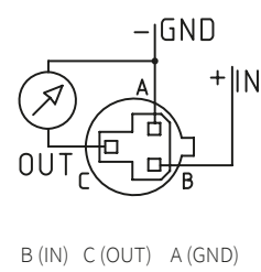
3 wire
