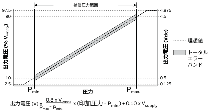
図 4. MIPシリーズ用 TEBの構成要素
