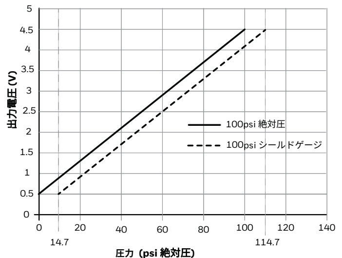
図3. 絶対圧 VS シールドゲージ圧
