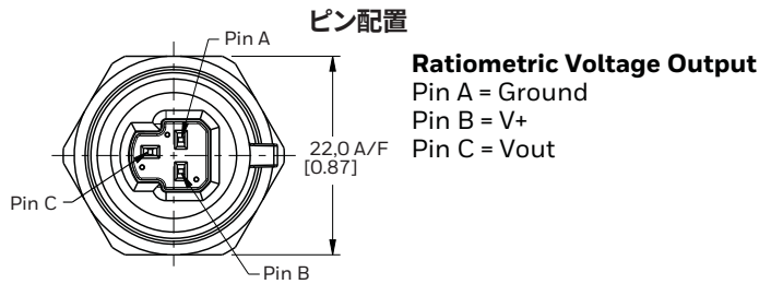
図 5. 取付け寸法 (参照のみ, MM)
