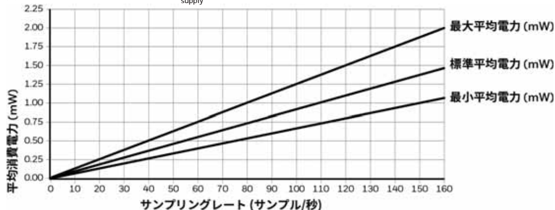
図 4. 平均消費電力VSサンプリングレート1.8V supply 時
