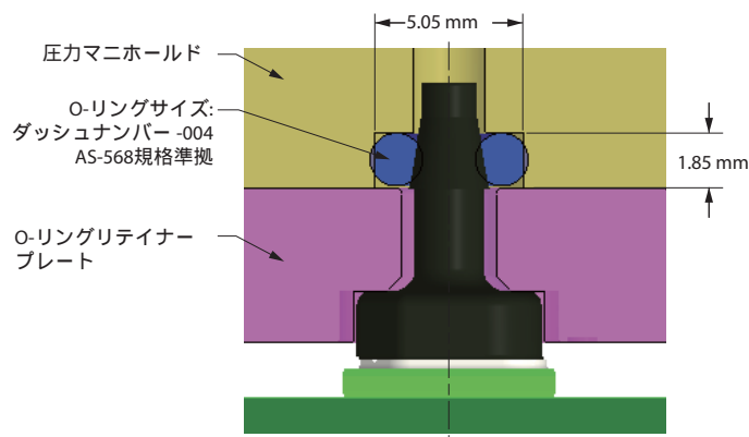
AN 圧力ポート
