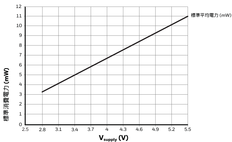
図6. アナログ出力バージョン標準消費電力
