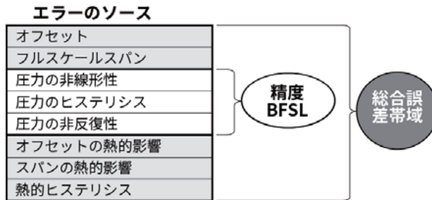
図 1. 総合誤差帯域 (トータルエラーバンドまたはTEB)
