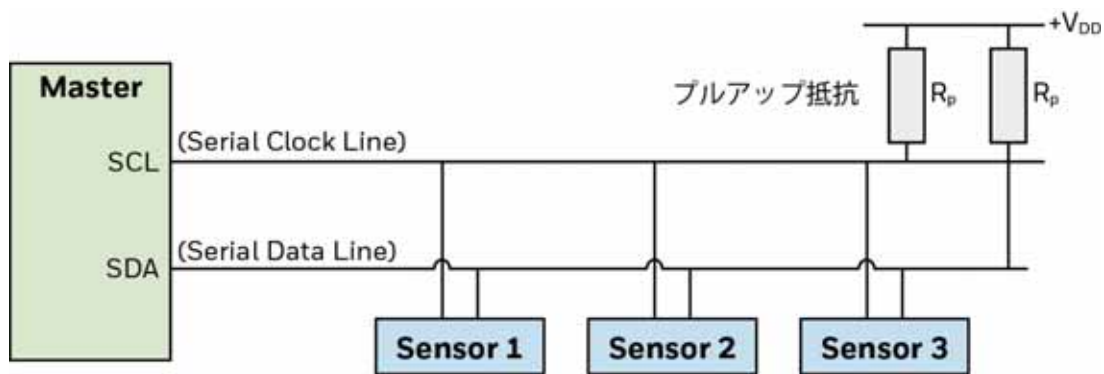
図 16. I 2 C バス構成
