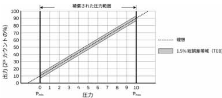
図 2. 伝達関数 (デジタル出力バージョン)
