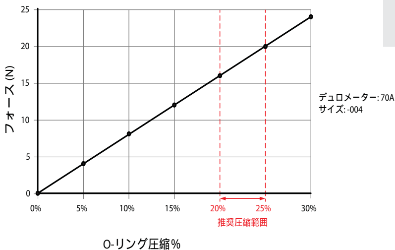
図20. フォース VS O-リング 圧縮%
