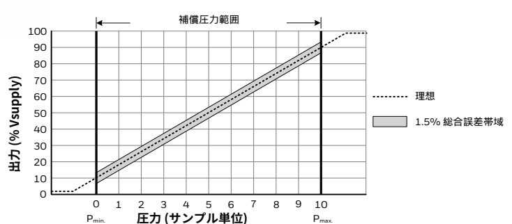
図 3. 伝達関数 (アナログ出力バージョン)
